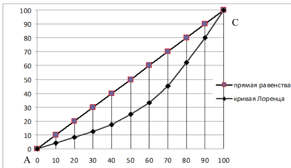
Рисунок 1 – Кривая Лоренца
